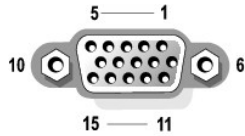
图 B-6. 视频连接器的插针编号
