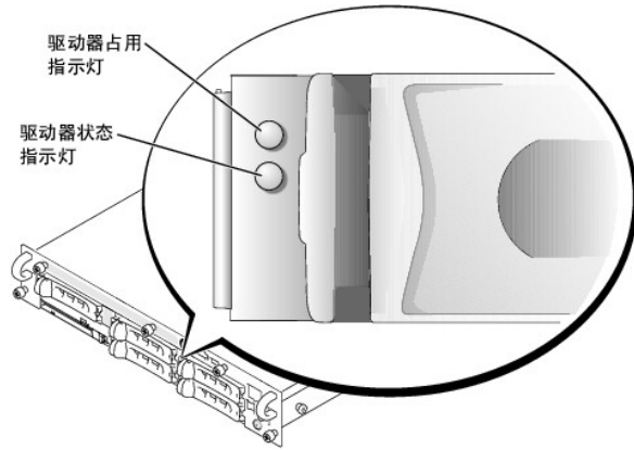
图 1-3. SCSI 硬盘驱动器指示灯
