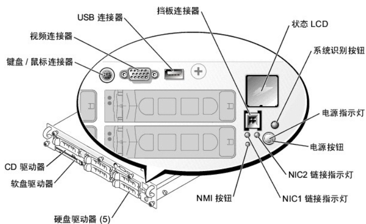
图 1-2. 前面板部件
