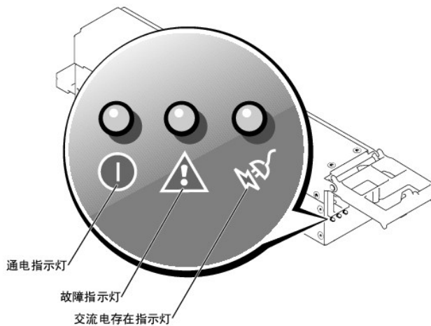
图1-5. 电源设备指示灯
