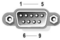
图 B-3. 串行端口的插针编号
