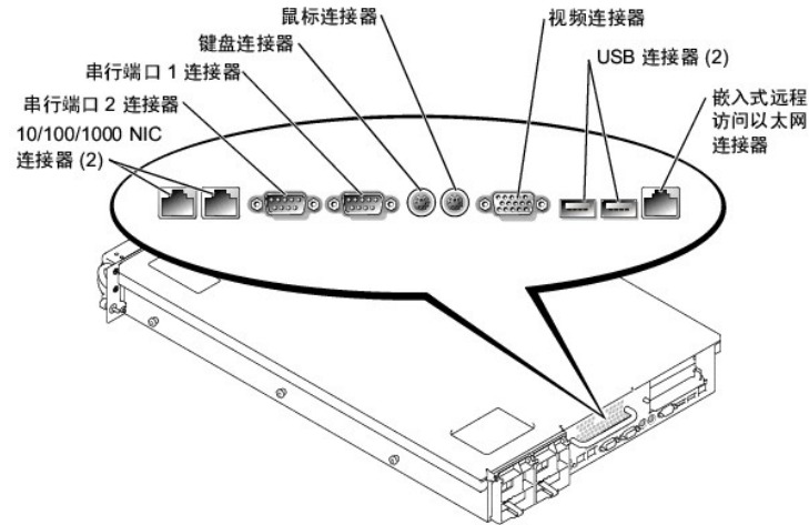
图 B-1. 背面板 I/O 端口和连接器
