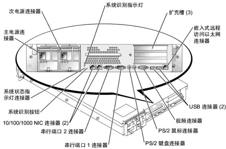
图1-4. 背面板部件
