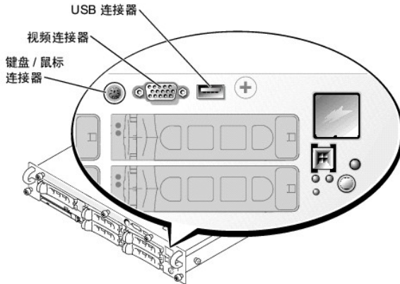
图 B-2. 前面板 I/O 端口和连接器
